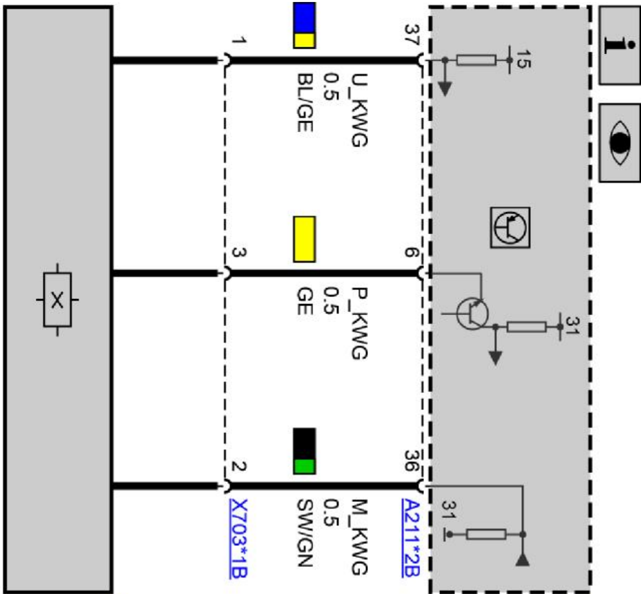
B6214a 曲轴传感器
